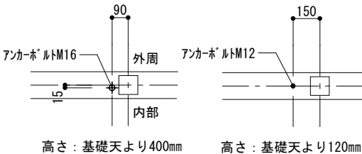
ホールダウン用アンカーボルト配置
